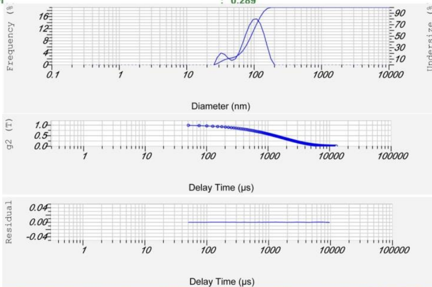
نمودار ۳- اندازه ذرات سامانه لیپوزومی حاوی عصاره‌ی Silybum marianum
